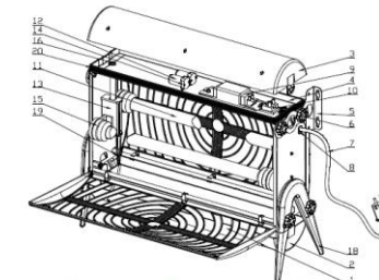
Rys. 1 Pułapka świetlna na owady DEAL-004 eco
