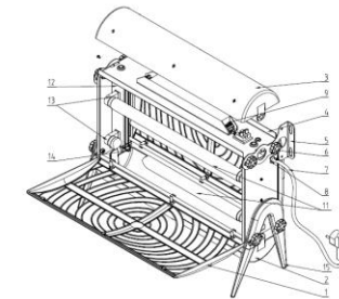
Rys. 1 Pułapka świetlna na owady DEAL-001eco
